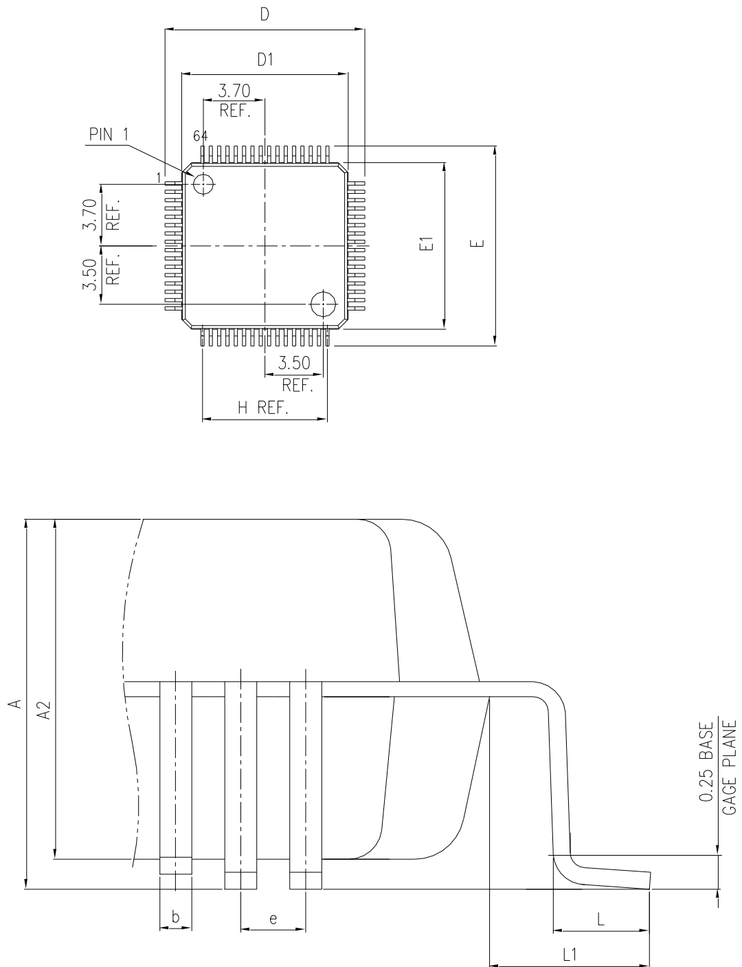
图 20 LQFP64 封装图
